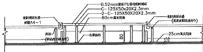
3 C向剖面圖 SCALE=1/60(A3 SIZE) SCALE=1/30(A1 SIZE)
